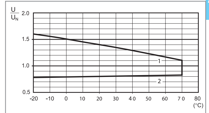
R 62 – 交流线圈工作范围对比环境温度 转换触点
