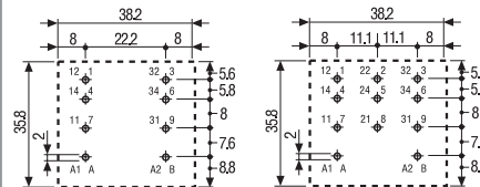
62.22 铜触点侧视图
