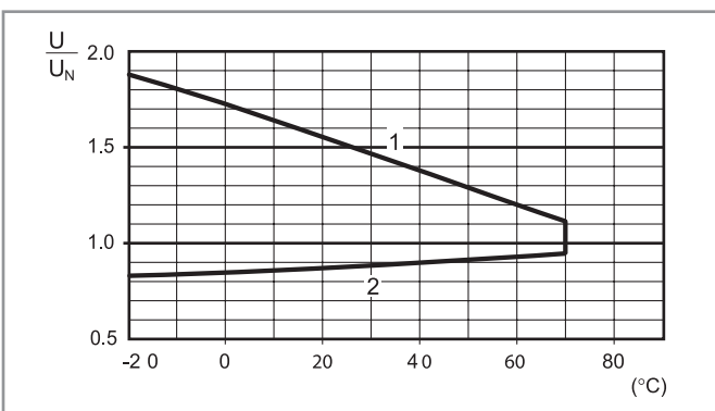
R 62 – 直流线圈工作范围对比环境温度 常开触点 - 磁偏吹型号
