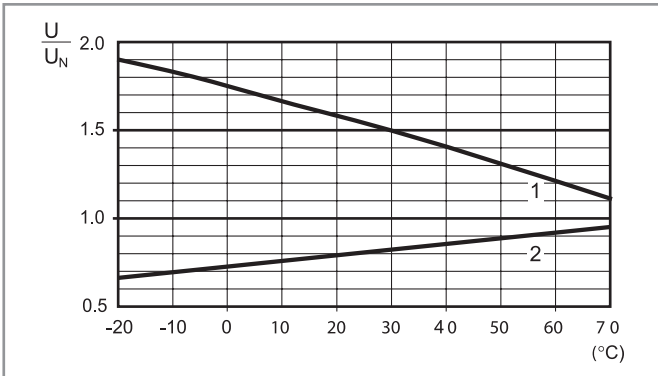
R 62 – 直流线圈工作范围对比环境温度 转换触点
