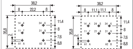
62.22-0300 铜触点侧视图
