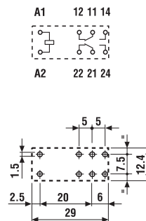
铜触点侧视图
