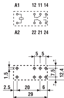
铜触点侧视图
